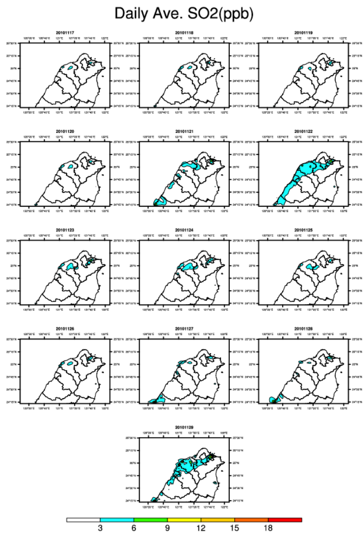
圖 B-11 (續) SO 2 地面等濃度圖
