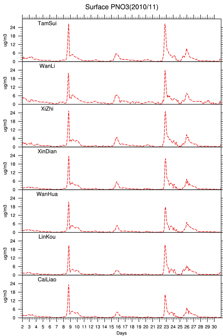
圖 B-7 NO 3 - 時間演變比較圖
