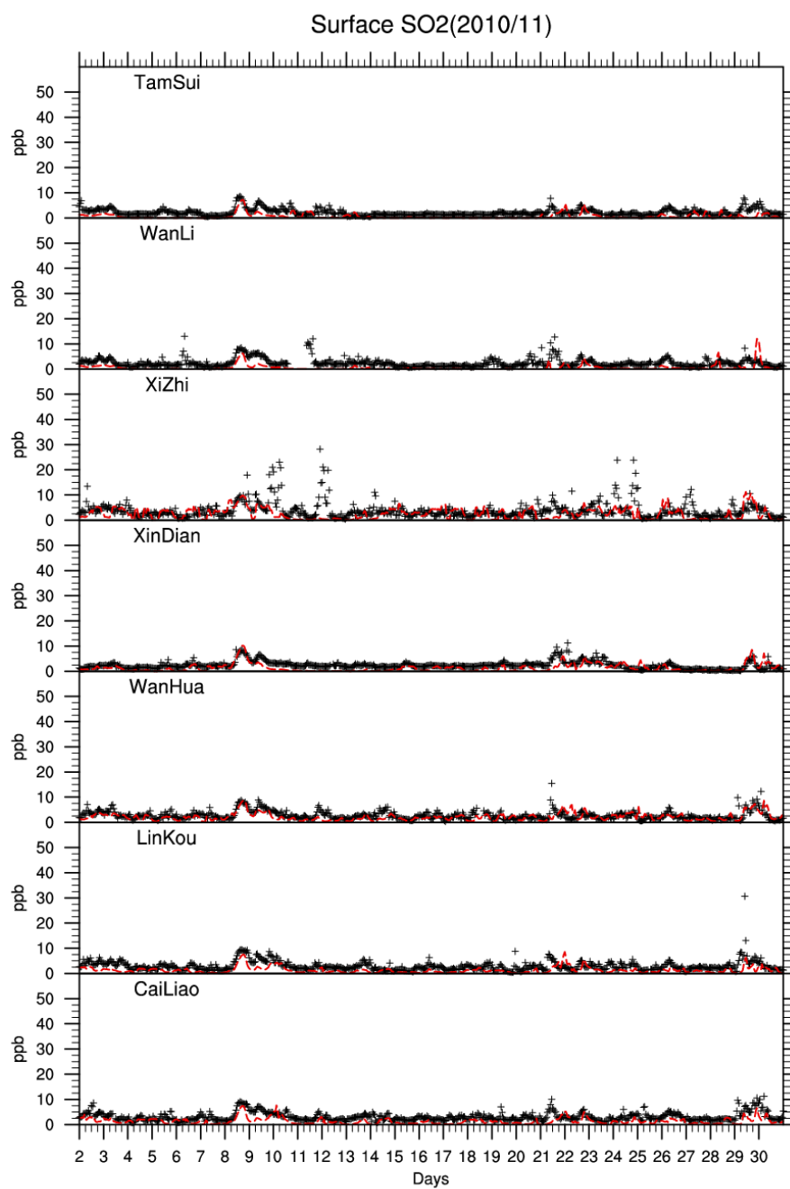
圖 B-4 SO 2 時間演變比較圖
