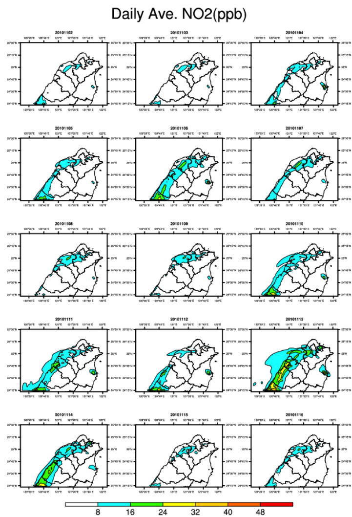
圖 B-12 NO 2 地面等濃度圖
