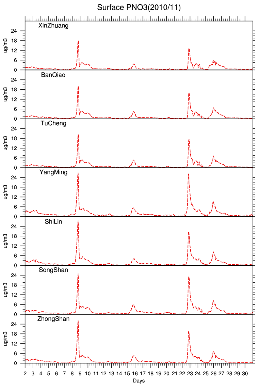
圖 B-7 (續) NO 3 - 時間演變比較圖
