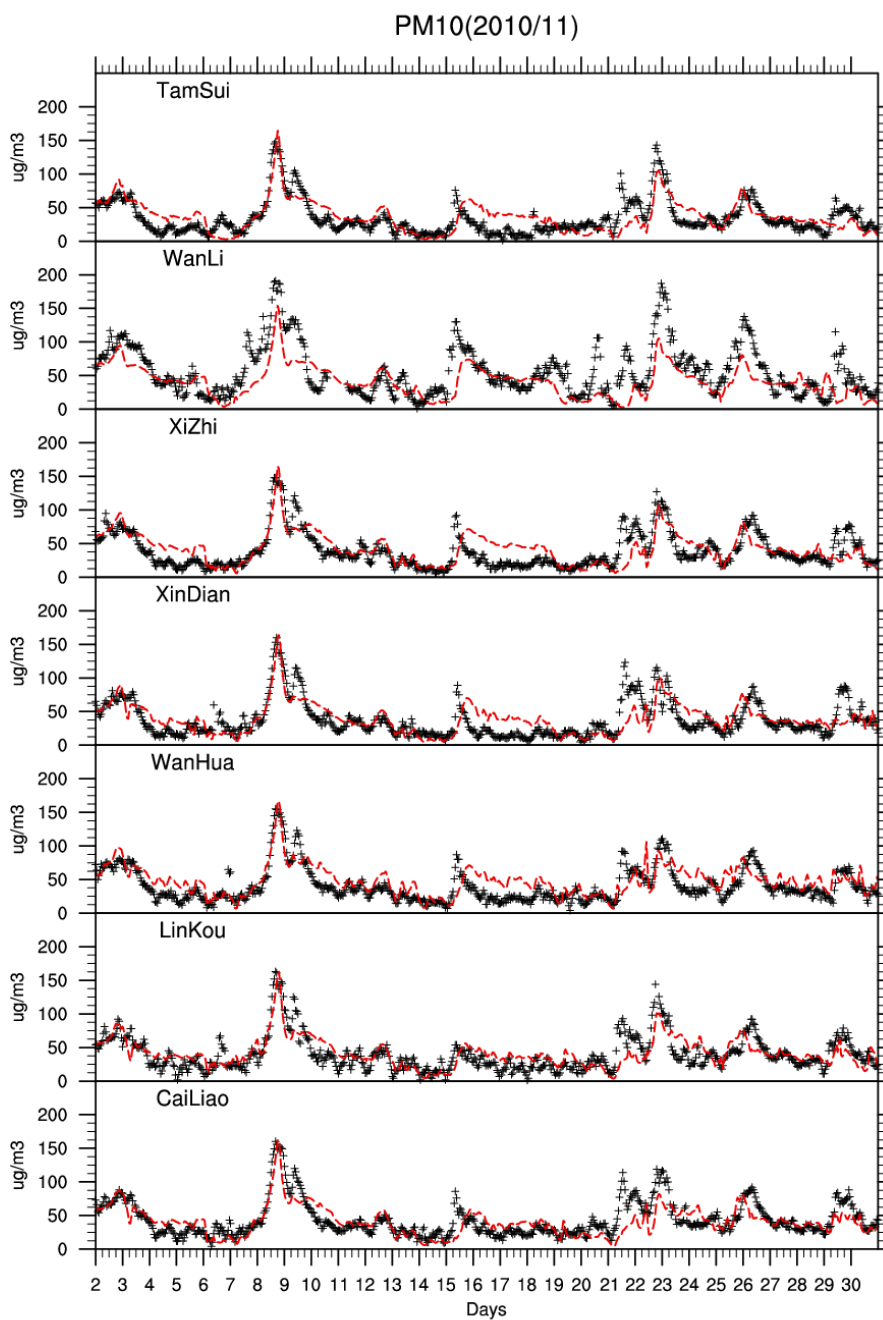
圖 B-2 PM 10 時間演變比較圖
