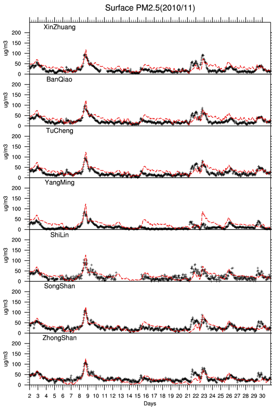
圖 B-3 (續) PM 2.5 時間演變比較圖
