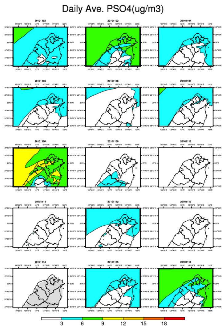
圖 B-13 SO 4 2- 地面等濃度圖
