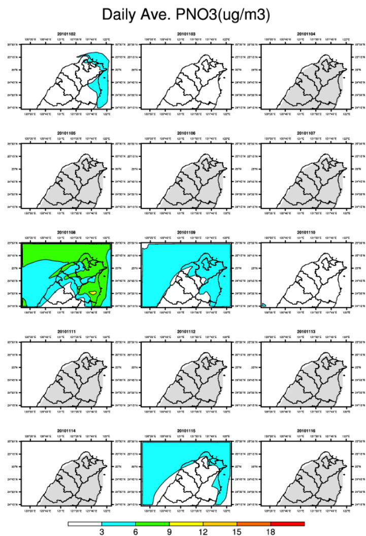
圖 B-14 NO 3 - 地面等濃度圖
