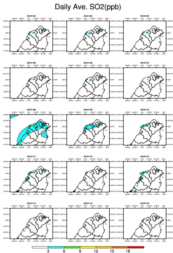
圖 B-11 SO 2 地面等濃度圖
