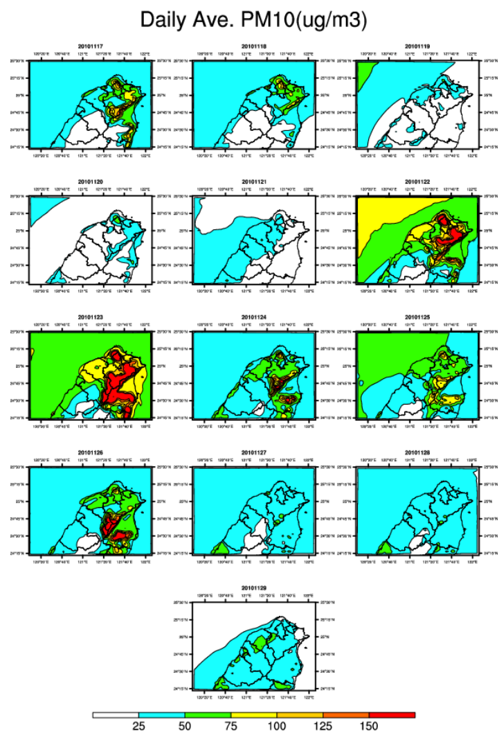
圖 B-9 (續) PM 10 地面等濃度圖
