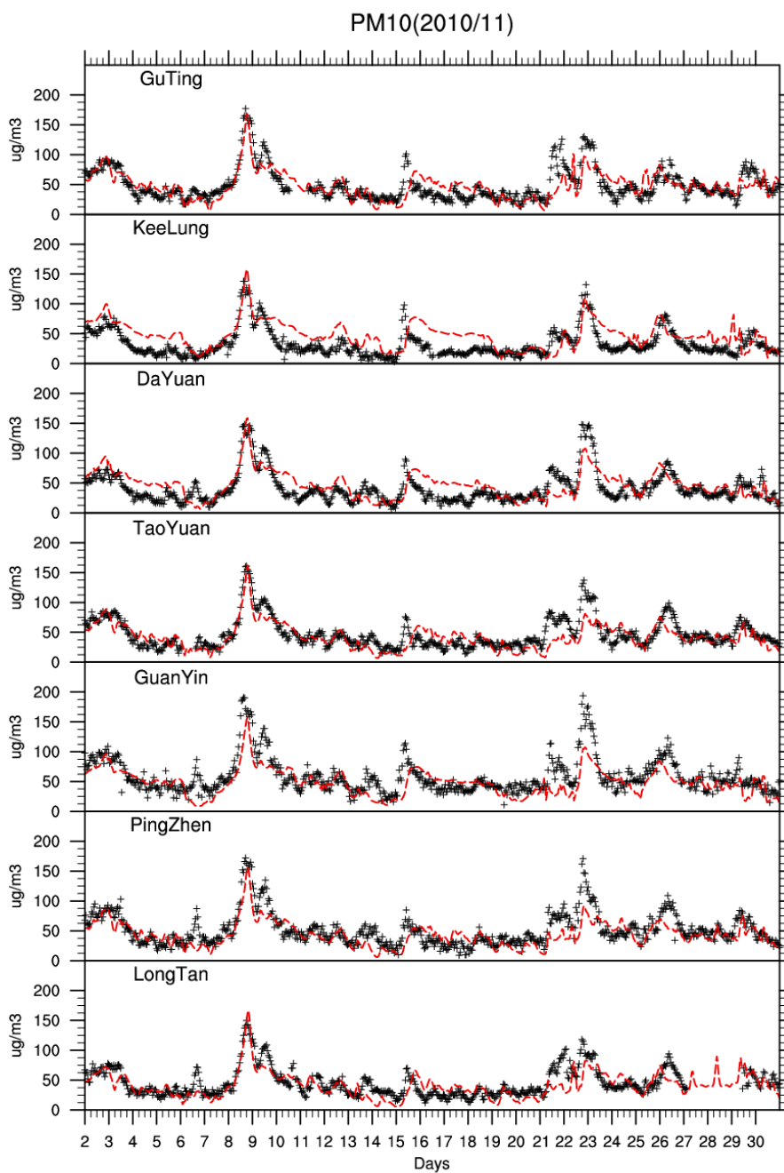
圖 B-2 (續) PM 10 時間演變比較圖
