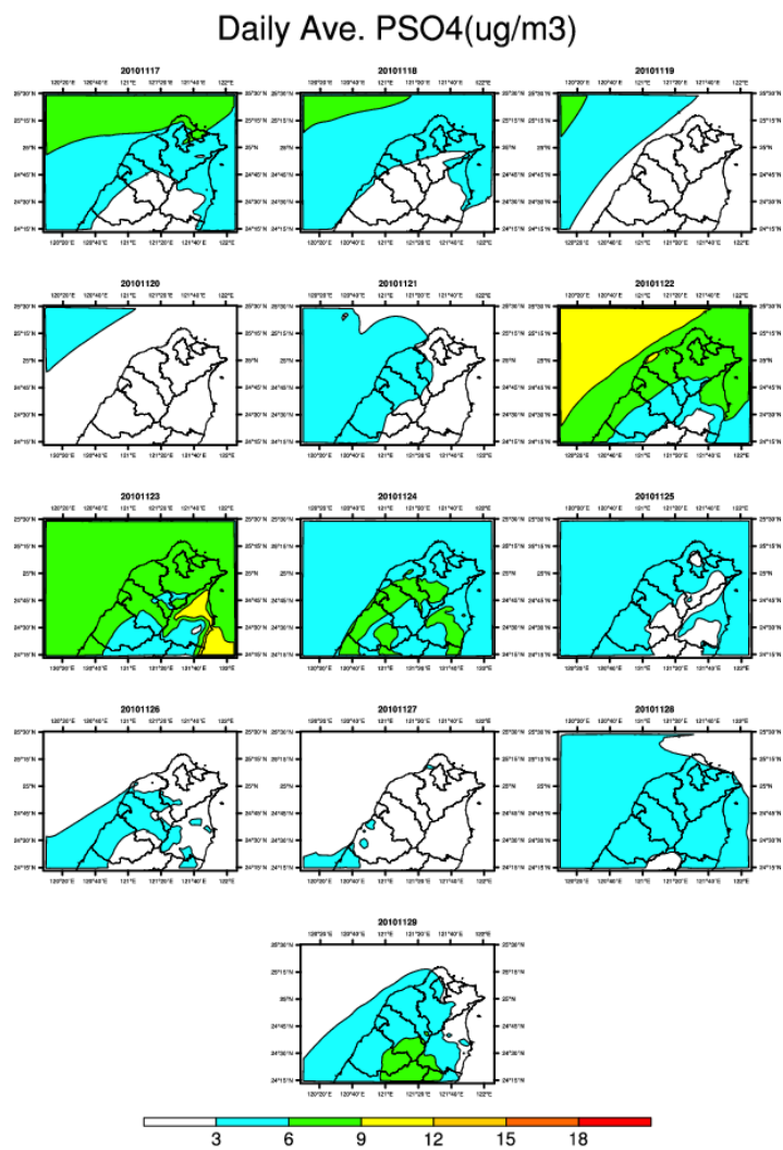
圖 B-13 (續) SO 4 2- 地面等濃度圖
