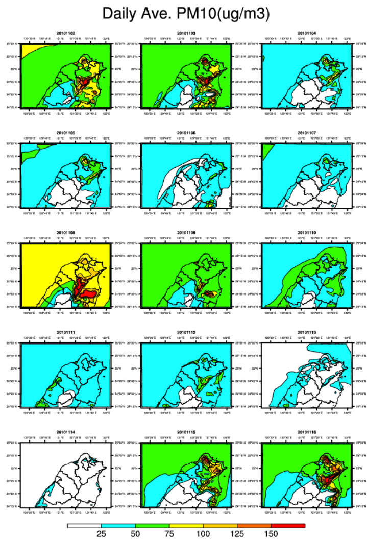
圖 B-9 PM 10 地面等濃度圖
