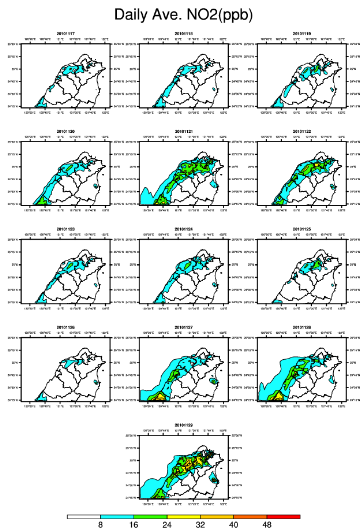
圖 B-12 (續) NO 2 地面等濃度圖
