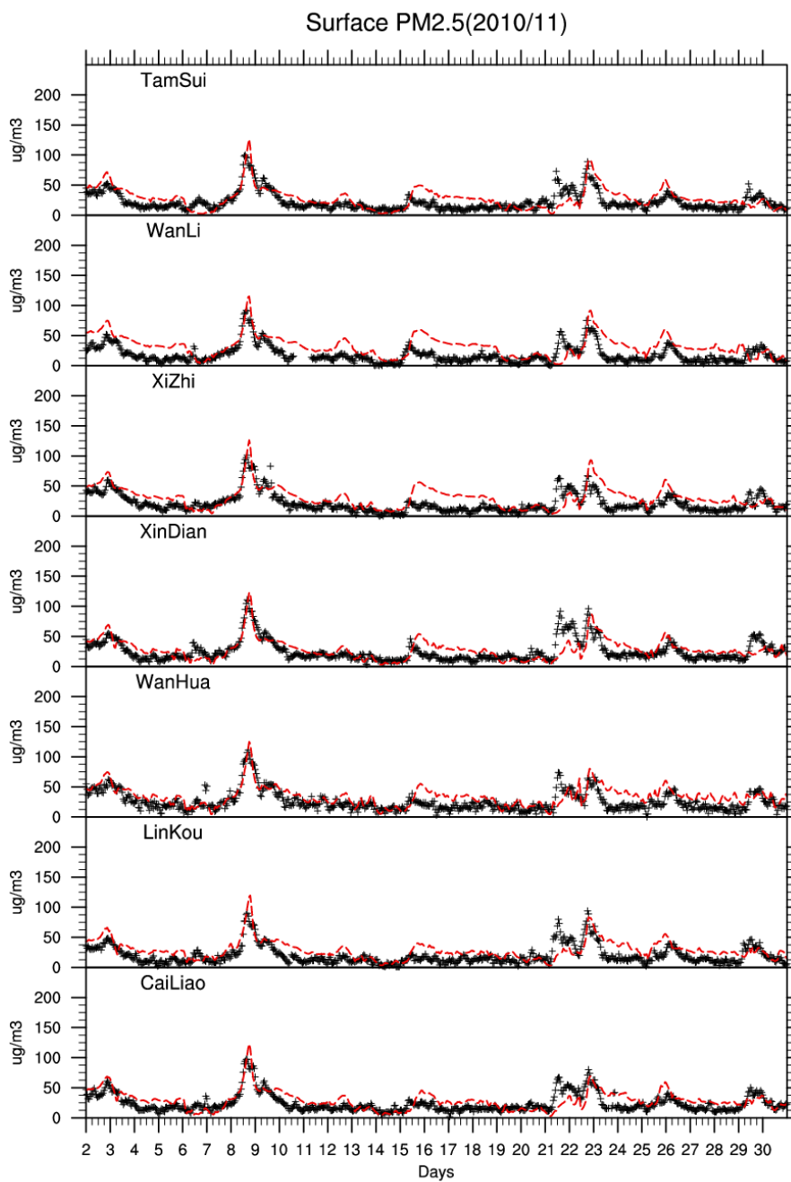
圖 B-3 PM 2.5 時間演變比較圖
