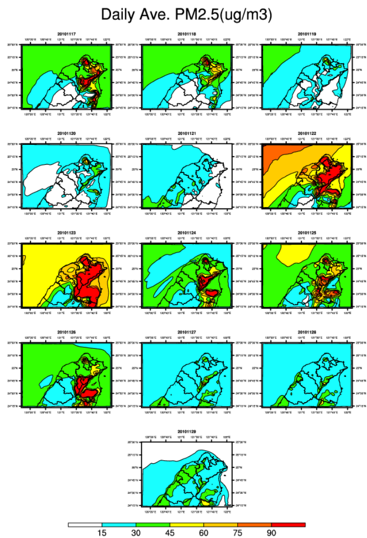
圖 B-10 (續) PM 2.5 地面等濃度圖
