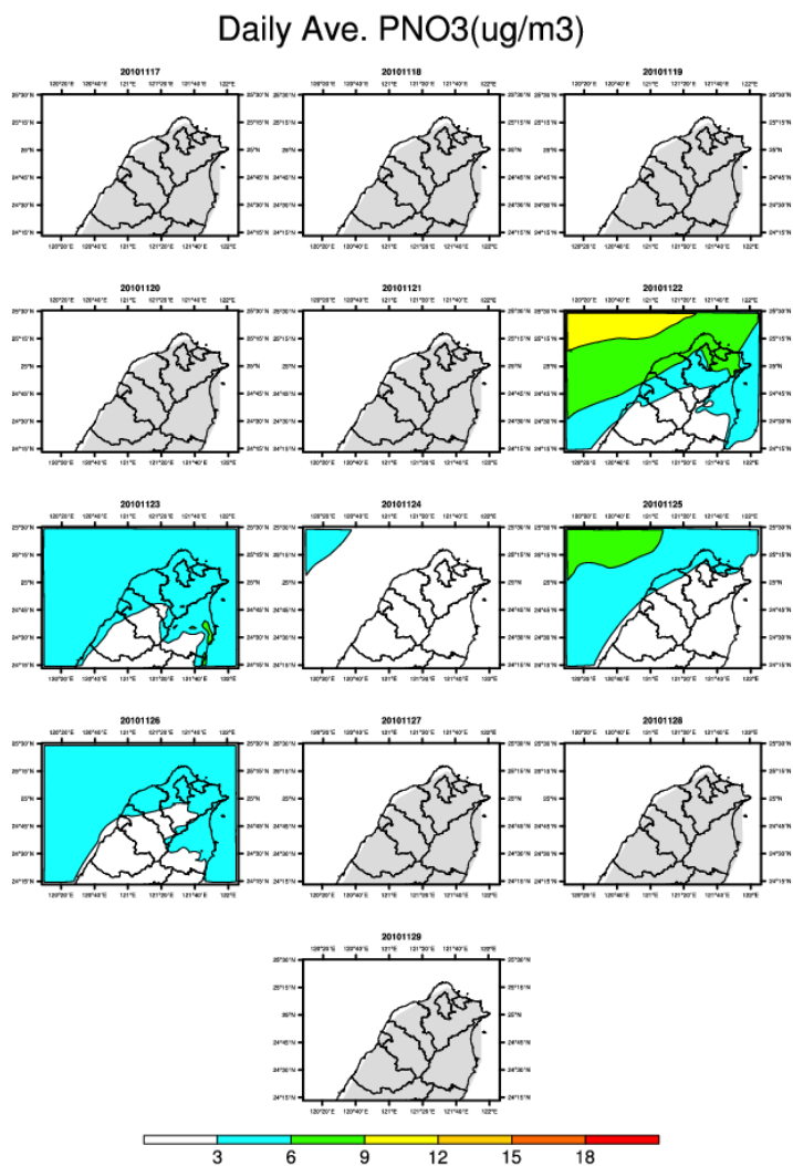
圖 B-14 (續) NO 3 - 地面等濃度圖
