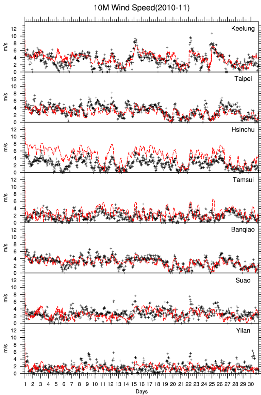
圖 B-15 風速時間演變比較圖
