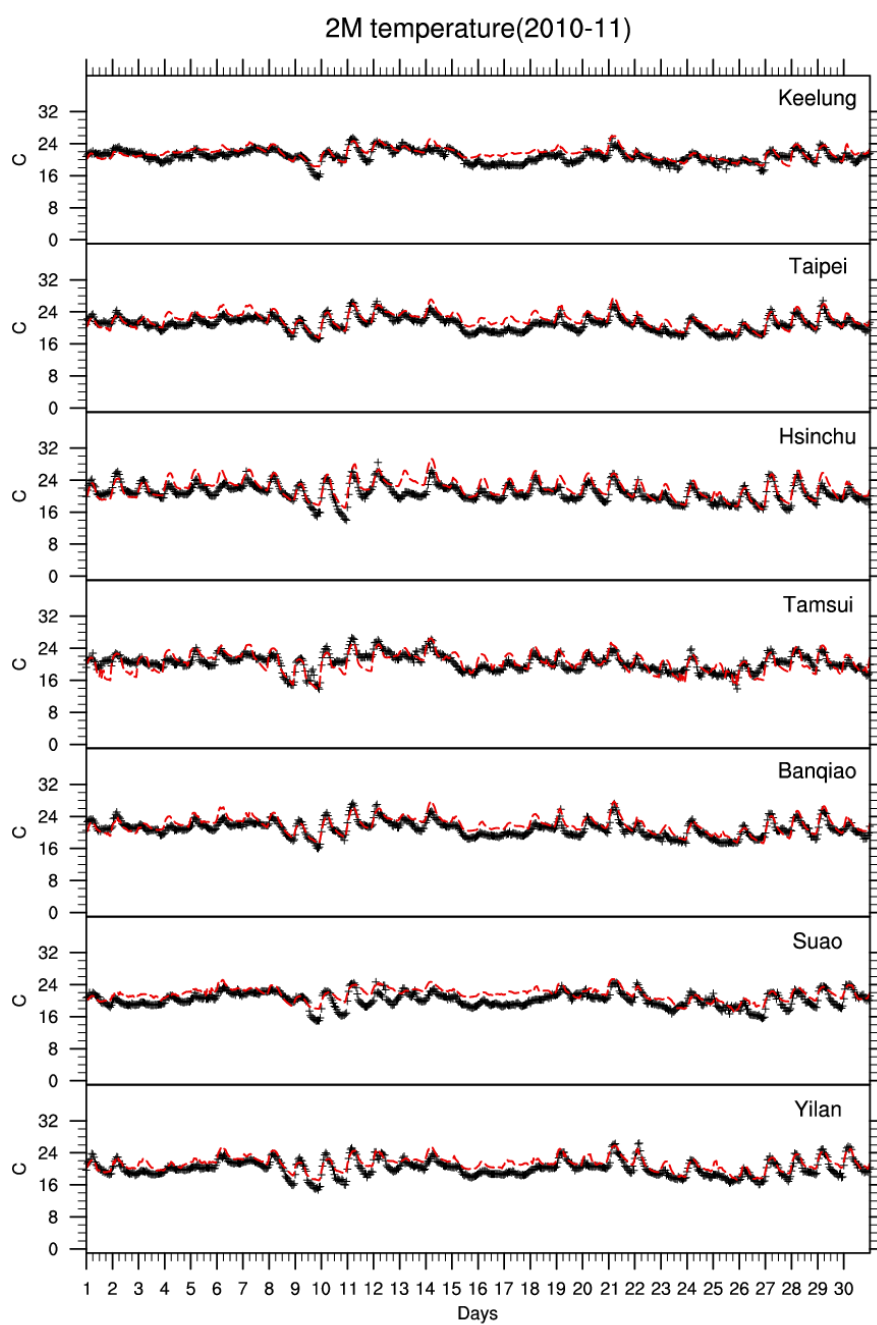
圖 B-16 溫度時間演變比較圖
