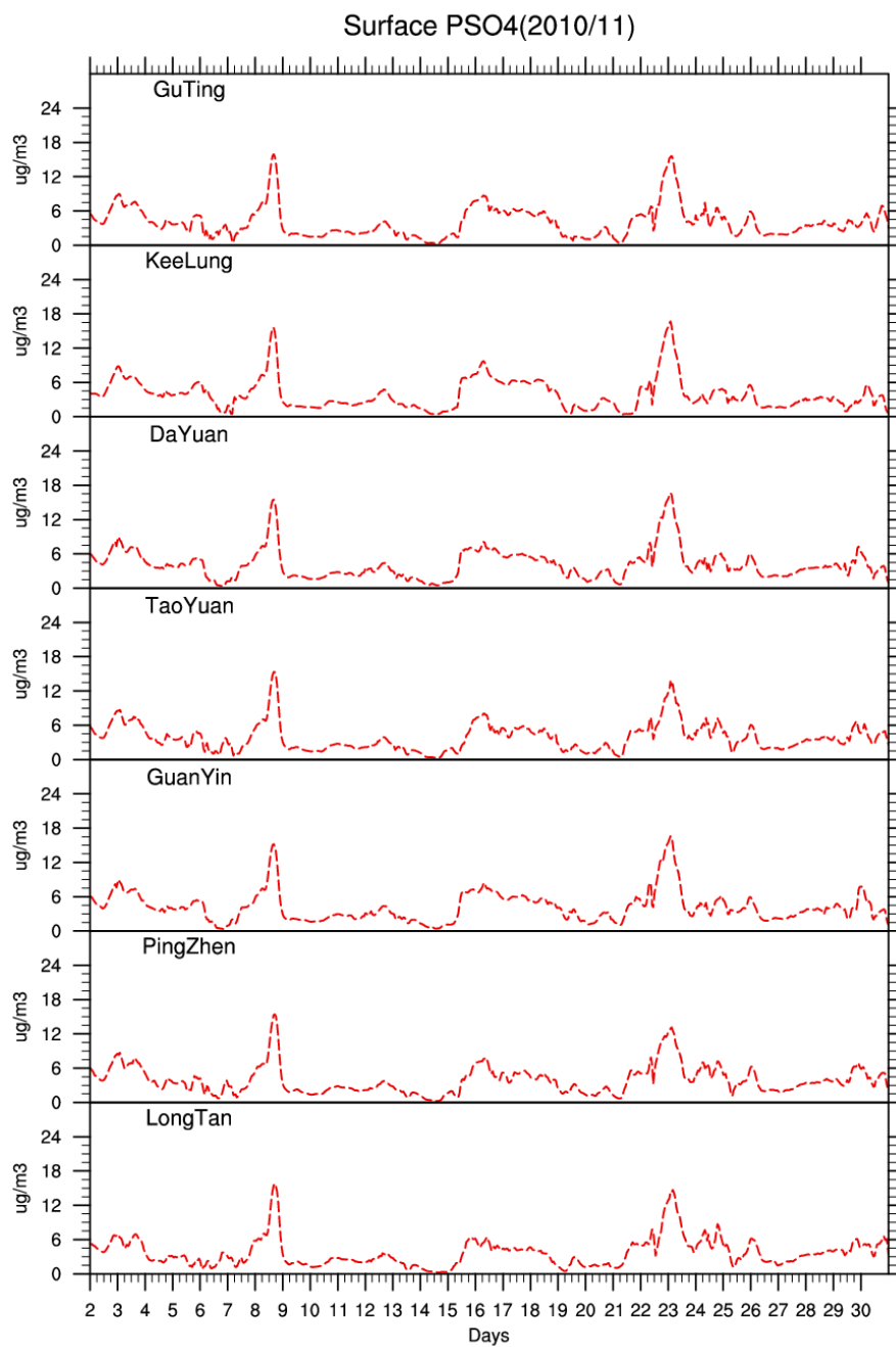
圖 B-6 (續) SO 4 2- 時間演變比較圖
