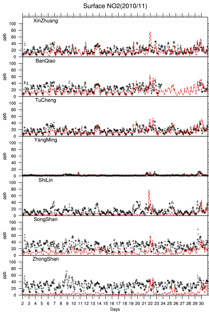
圖 B-5 (續) NO 2 時間演變比較圖
