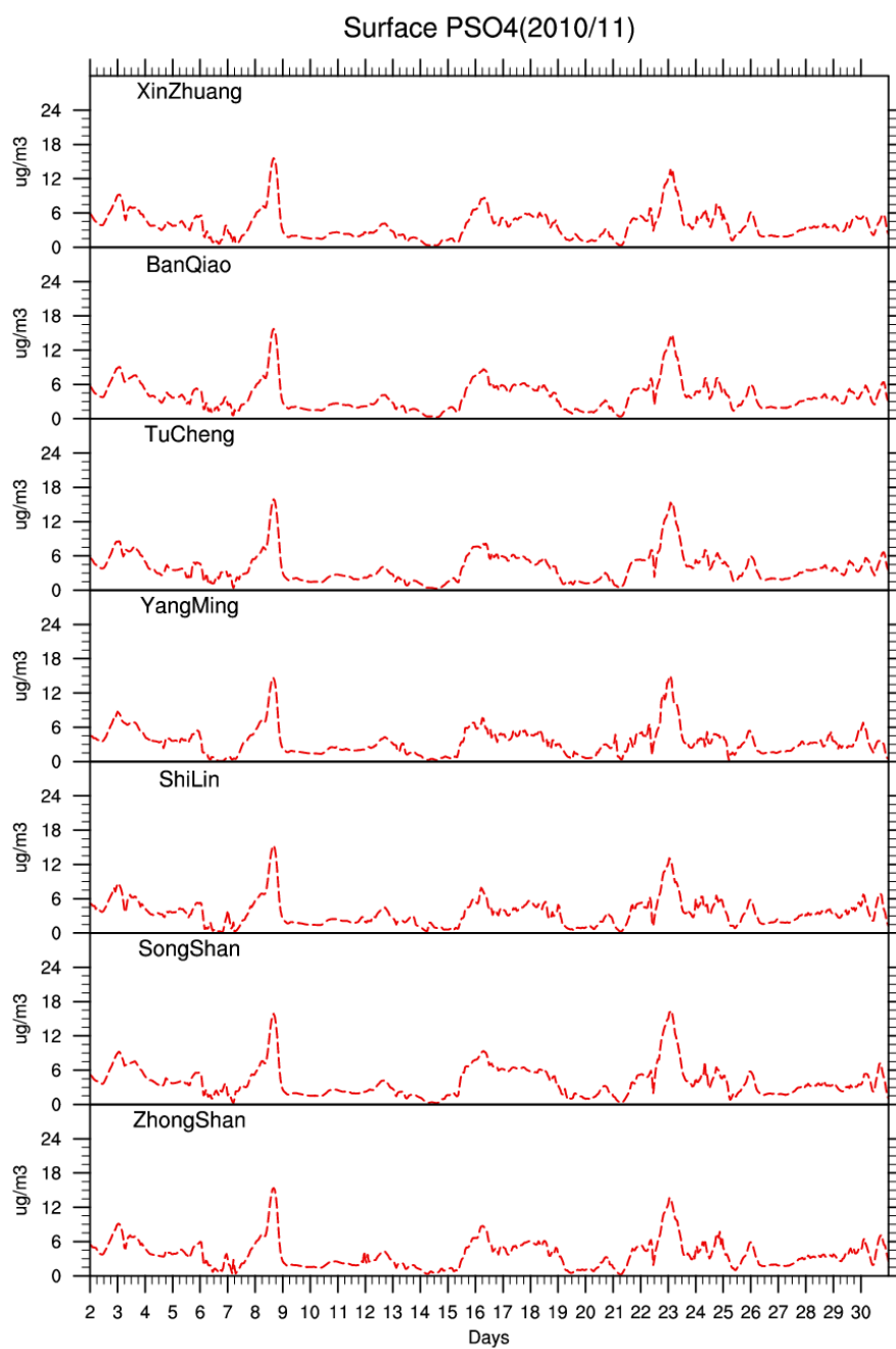
圖 B-6 (續) \text{SO}_4^{2-} 時間演變比較圖
