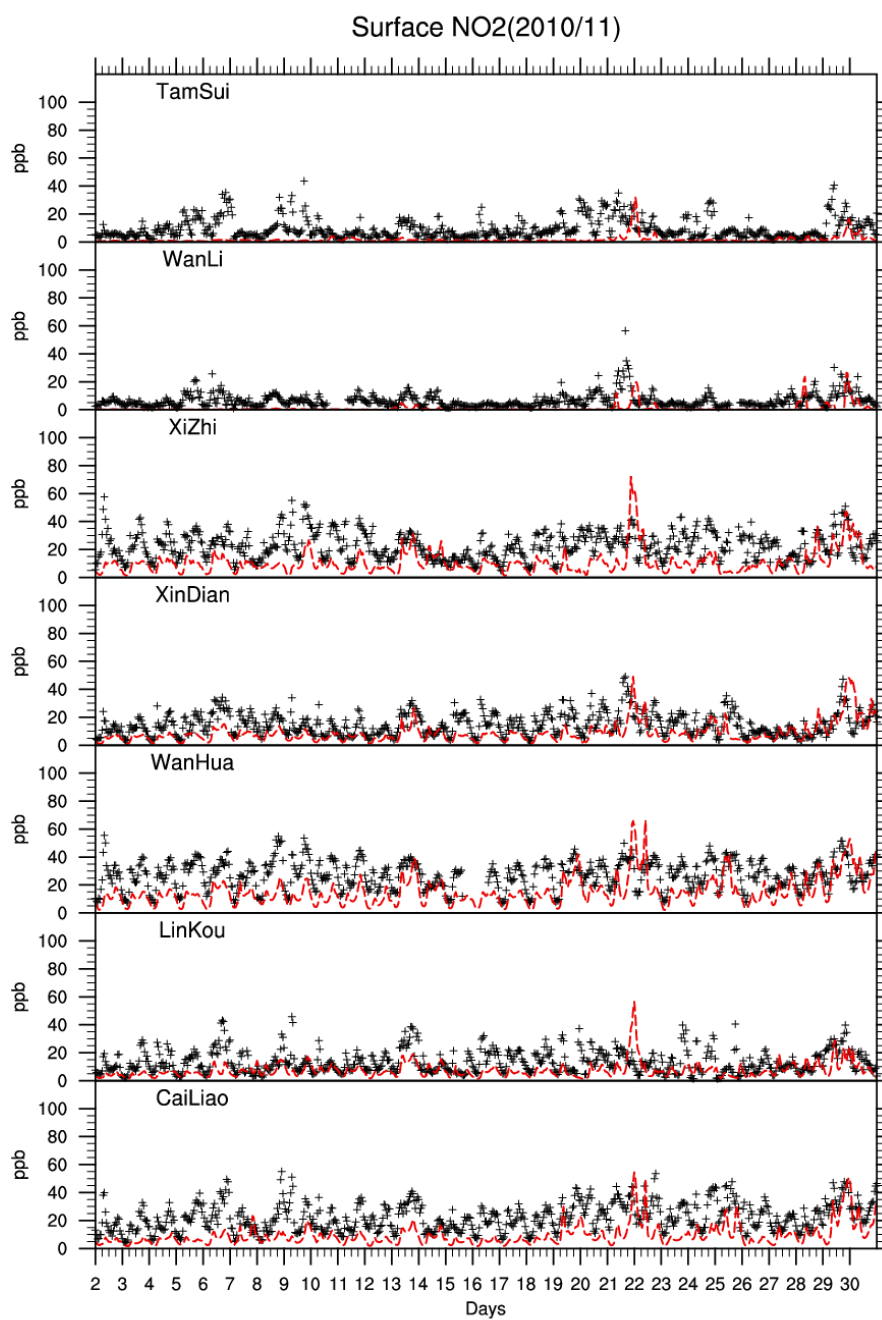
圖 B-5 NO 2 時間演變比較圖
