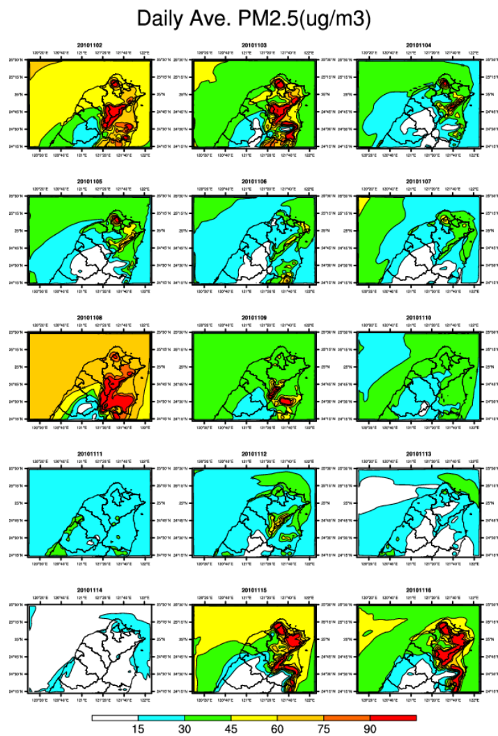
圖 B-10 PM 2.5 地面等濃度圖
