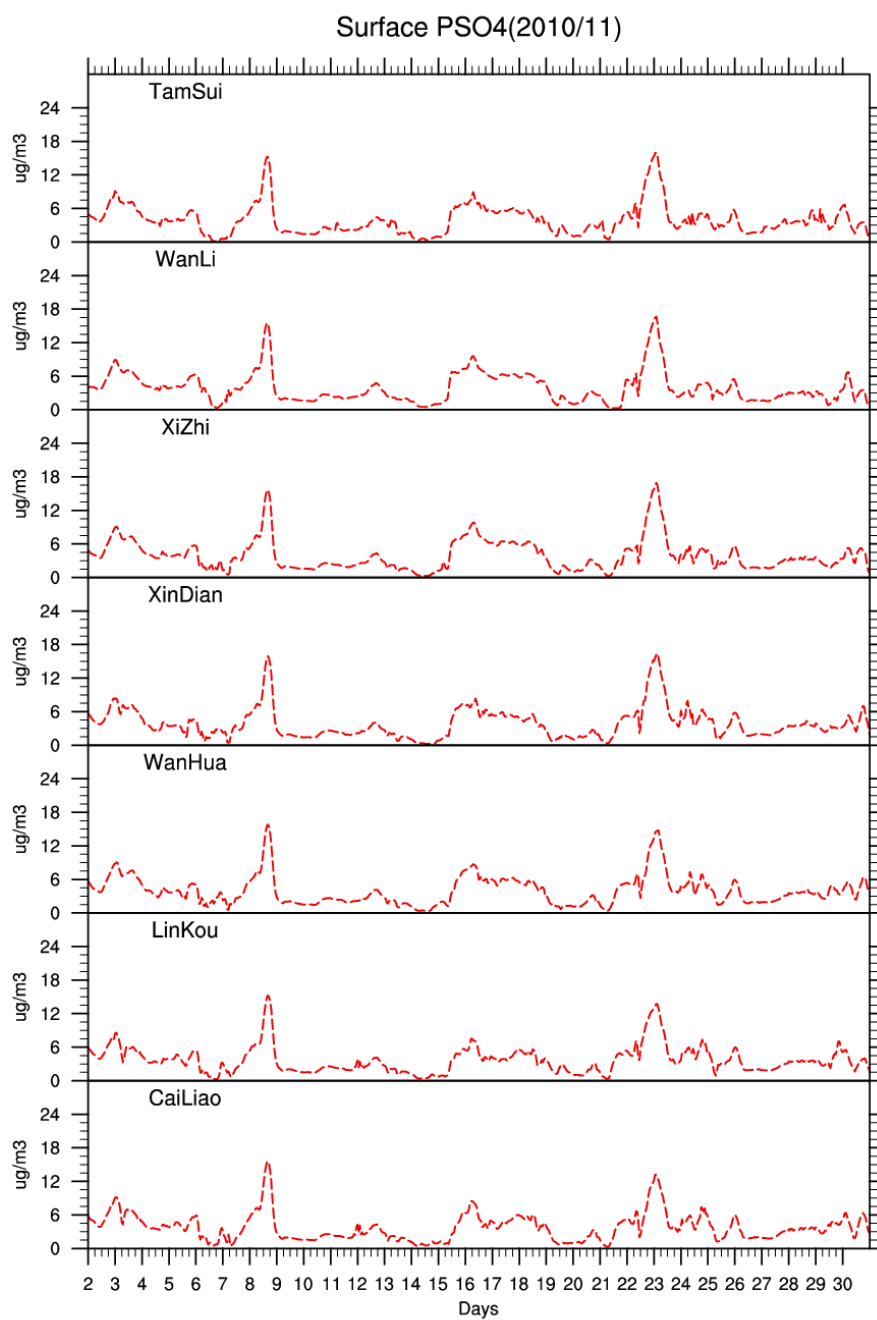
圖 B-6 \text{SO}_4^{2-} 時間演變比較圖
