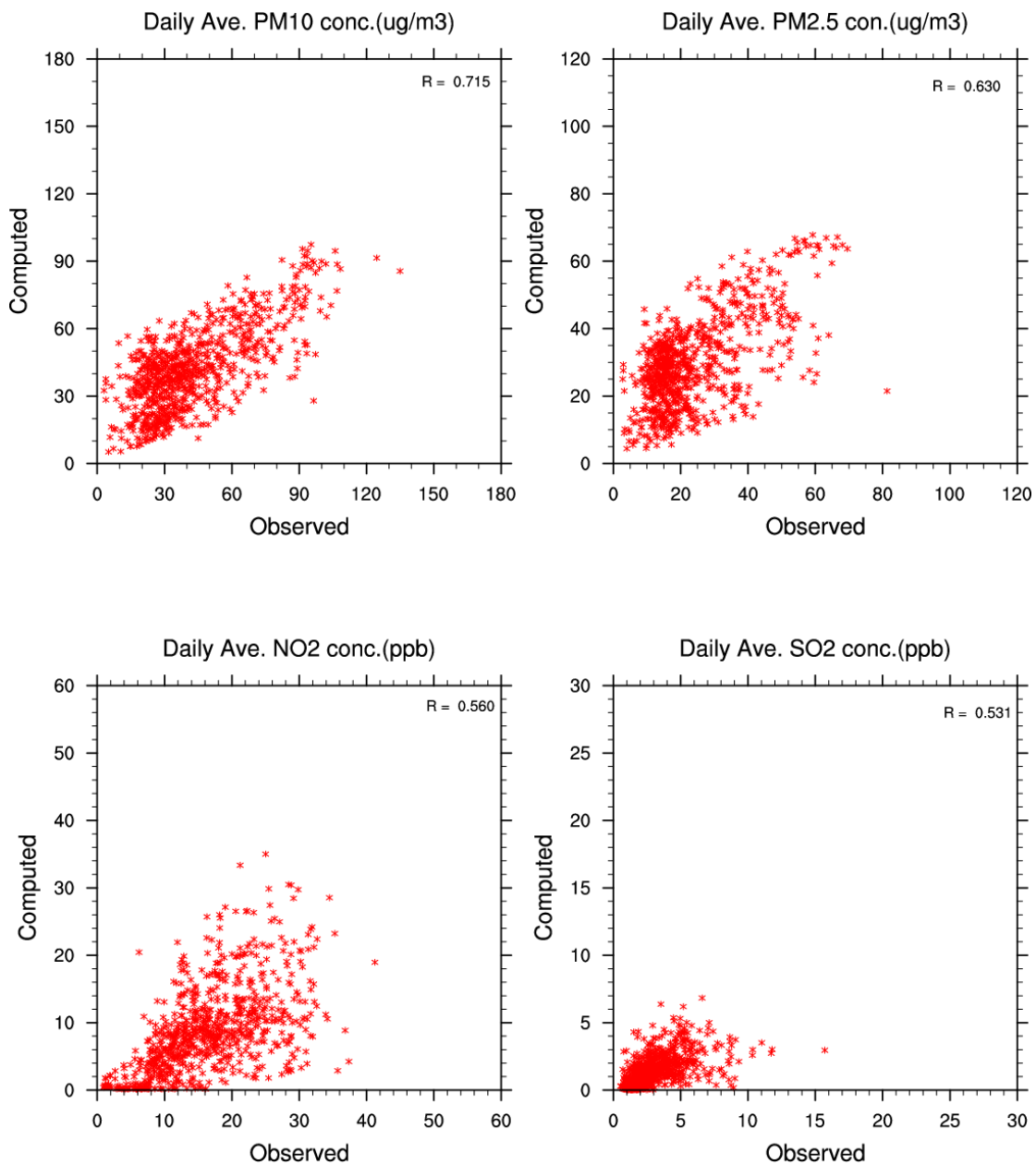
圖 B-8 PM 10 、PM 2.5 、NO 2 、SO 2 散布圖
