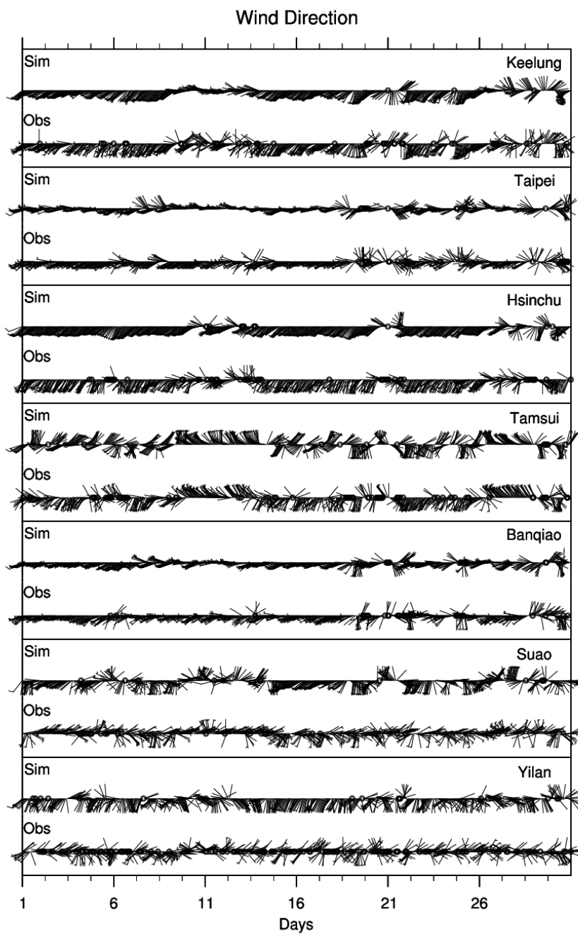
圖 B-17 風向時間演變比較圖
