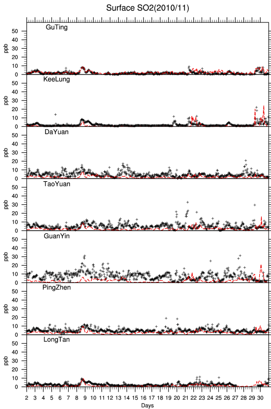
圖 B-4 (續) SO 2 時間演變比較圖
