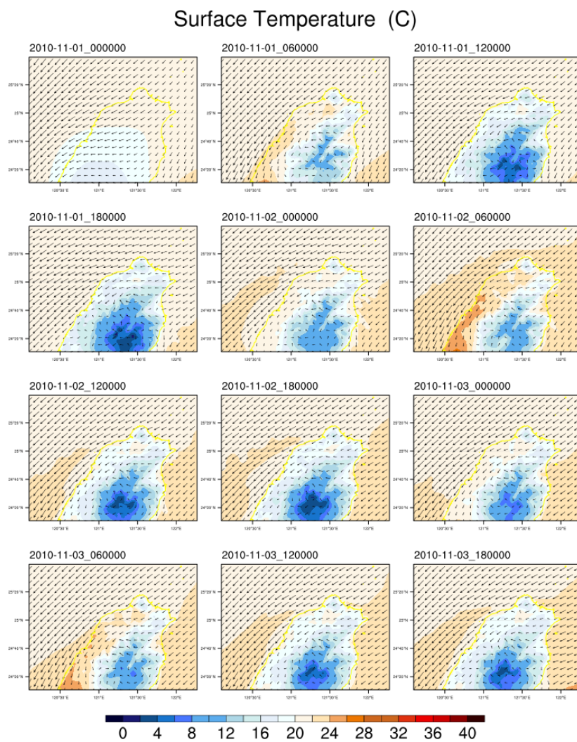
圖 B-20 平面風場分布圖
