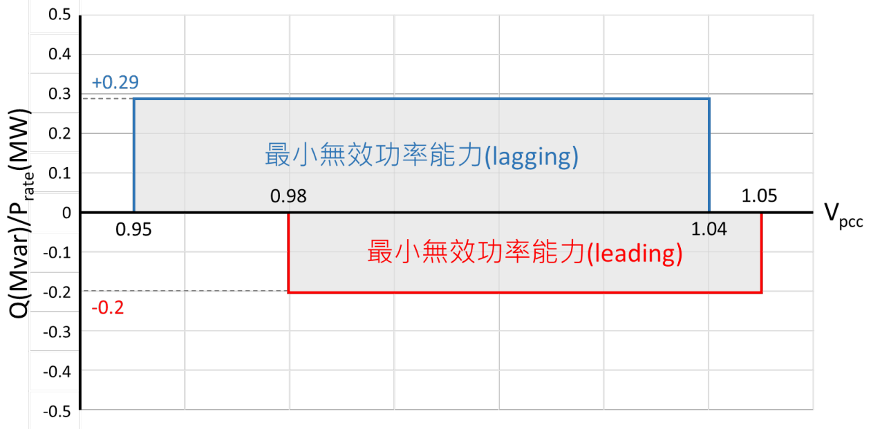
(a) 適用已完成遴選、競價及區塊開發3-1期之離岸風力發電設備
