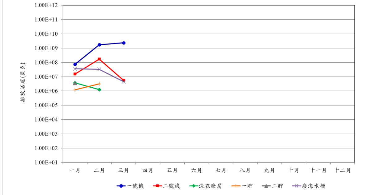
圖十一 核一廠各廢液排放源-總排放活度統計圖
