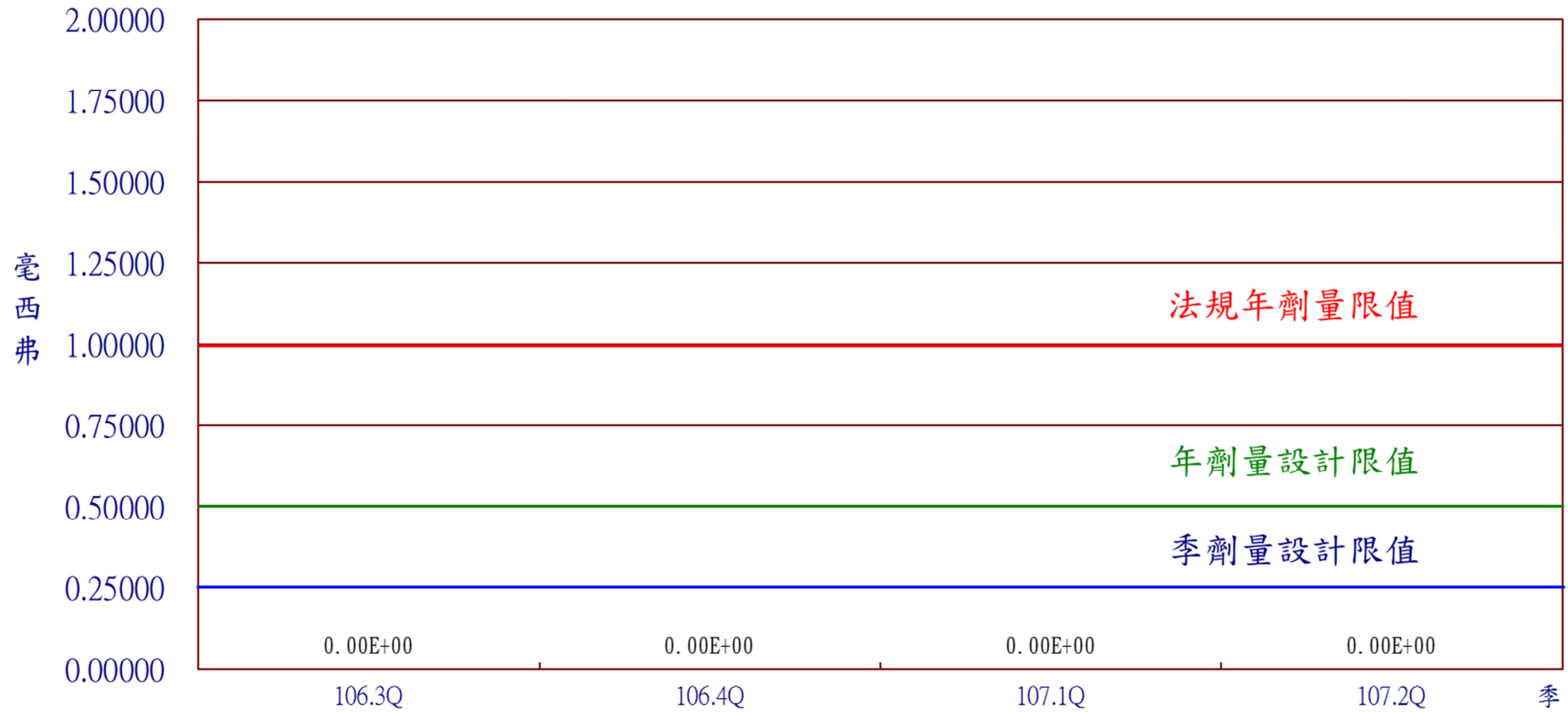
圖16 核能二廠107年第2季民眾最大個人全身劑量
