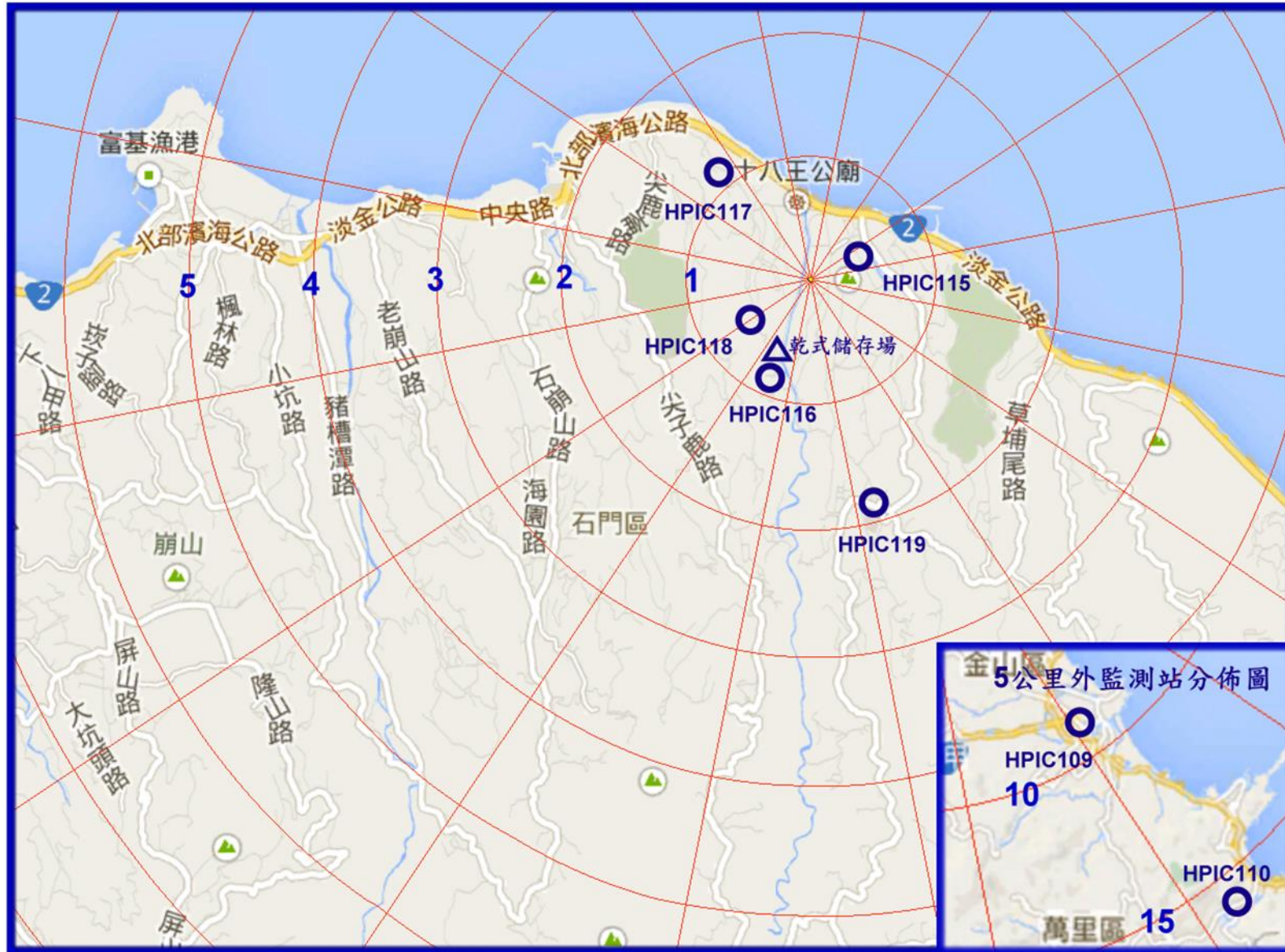
圖 3 核能一廠高壓游離腔監測站分佈圖
