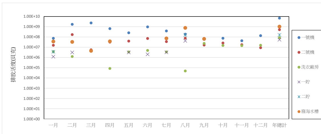
圖 12 112 年各廢水排放源總排放活度統計圖
