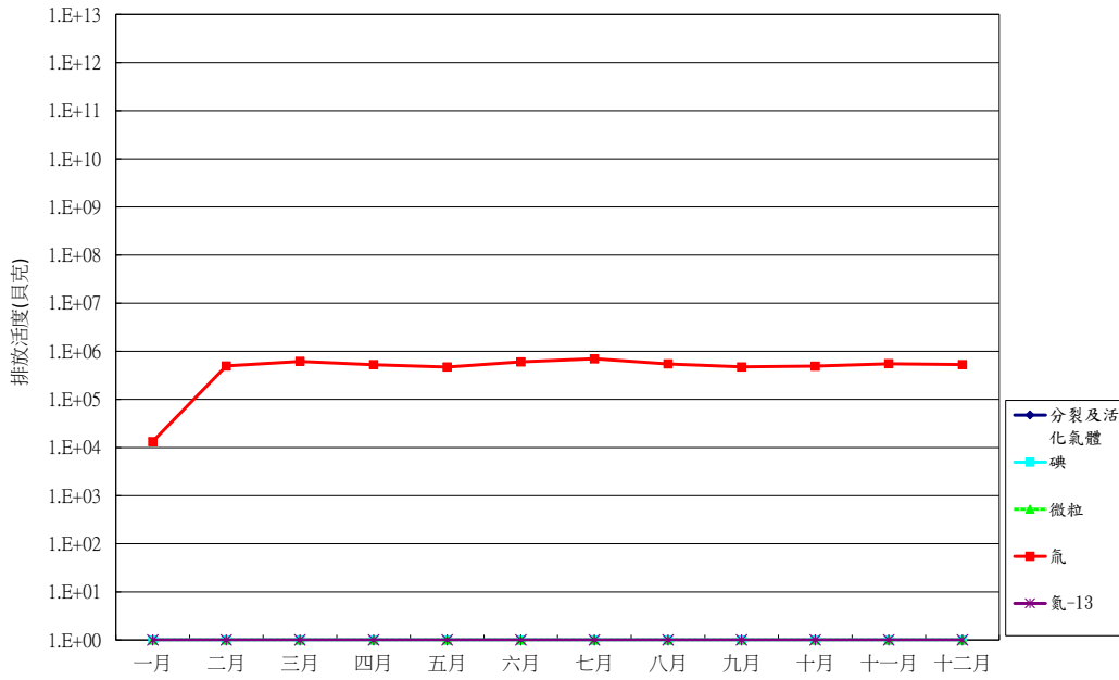
圖 7 112 年主煙囪放射性廢氣排放活度統計圖
