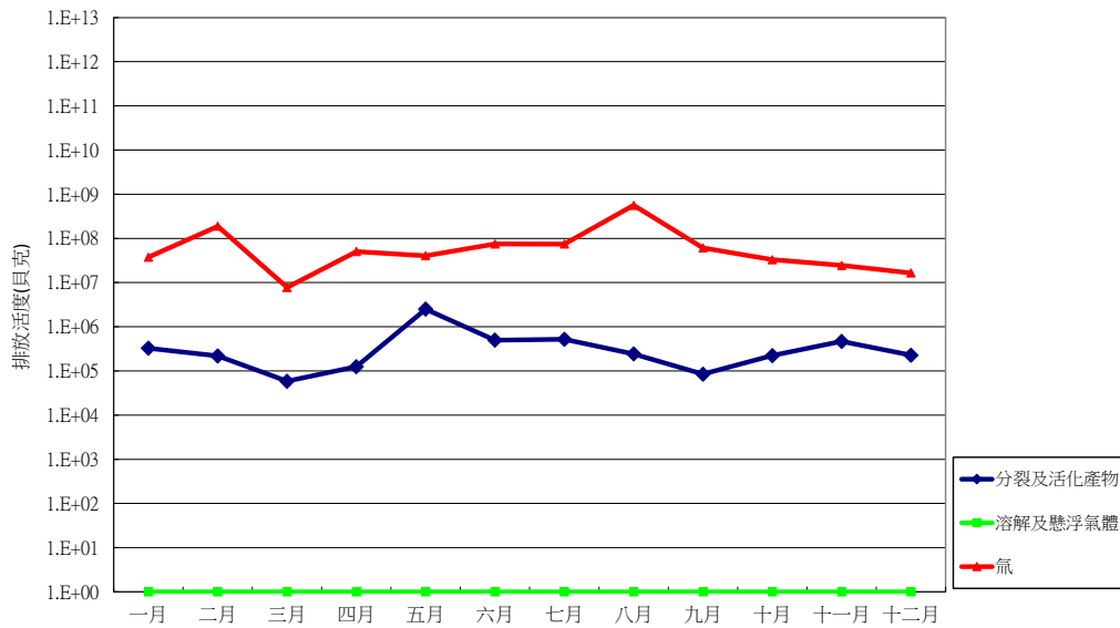
圖 11 112 年二號機放射性廢水排放活度統計圖
