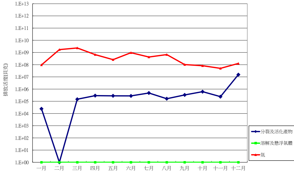
圖 10 112 年一號機放射性廢水排放活度統計圖
