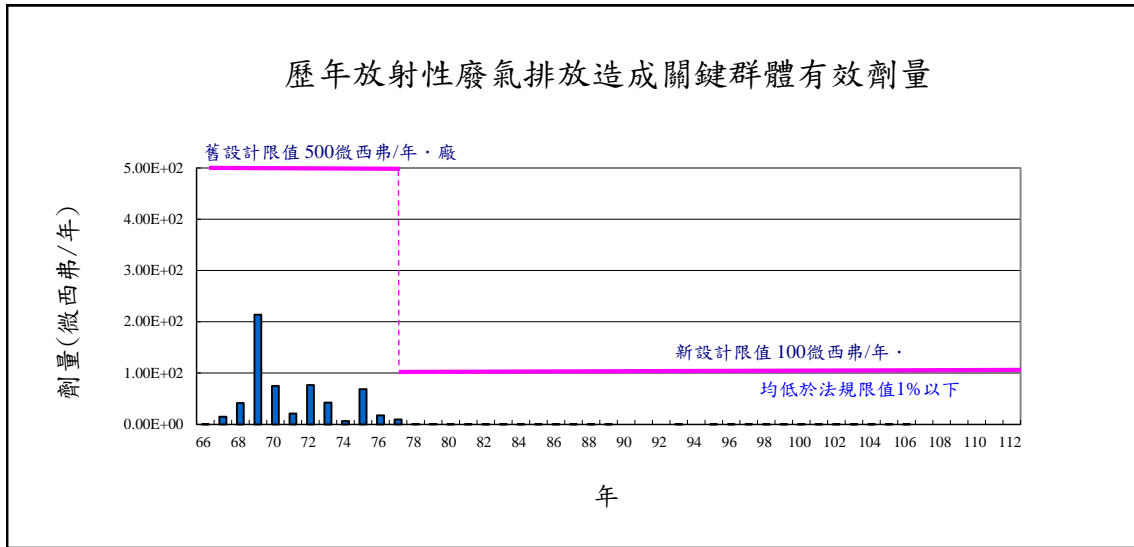
圖 14 歷年放射性廢氣排放造成關鍵群體有效劑量趨勢
