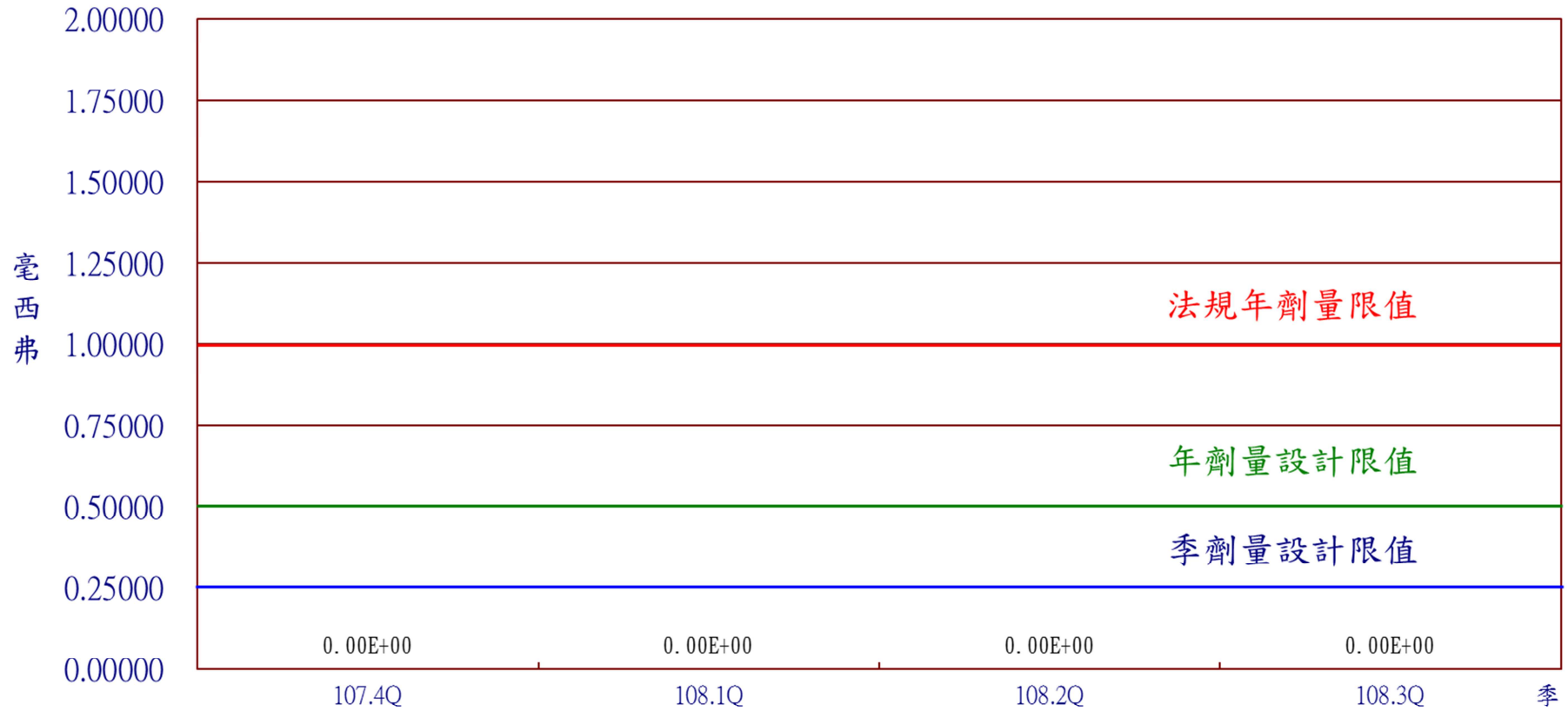
圖16 核能二廠108年第3季民眾最大個人全身劑量
