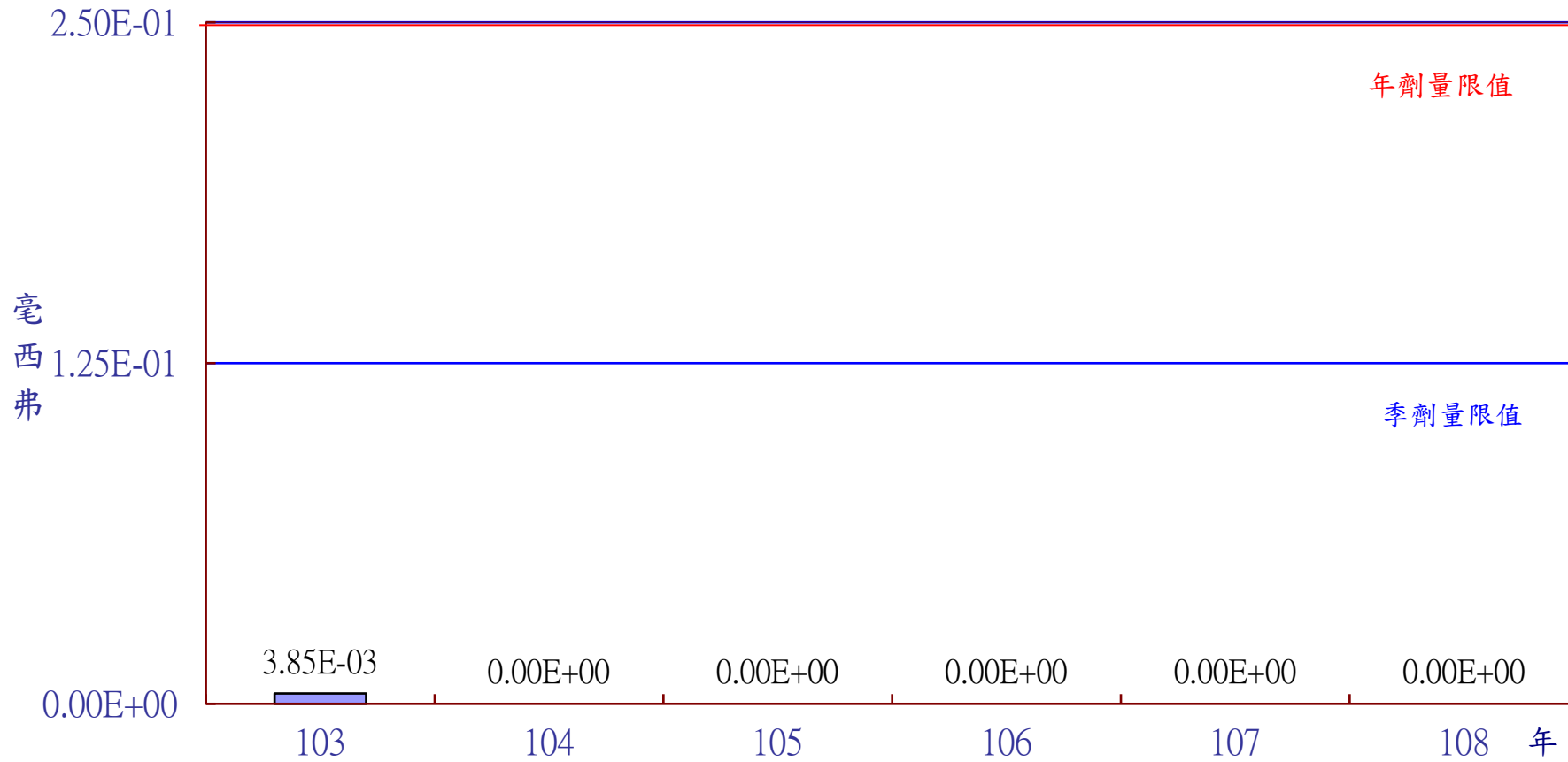
圖5 低放貯存場108年民眾最大個人全身劑量
