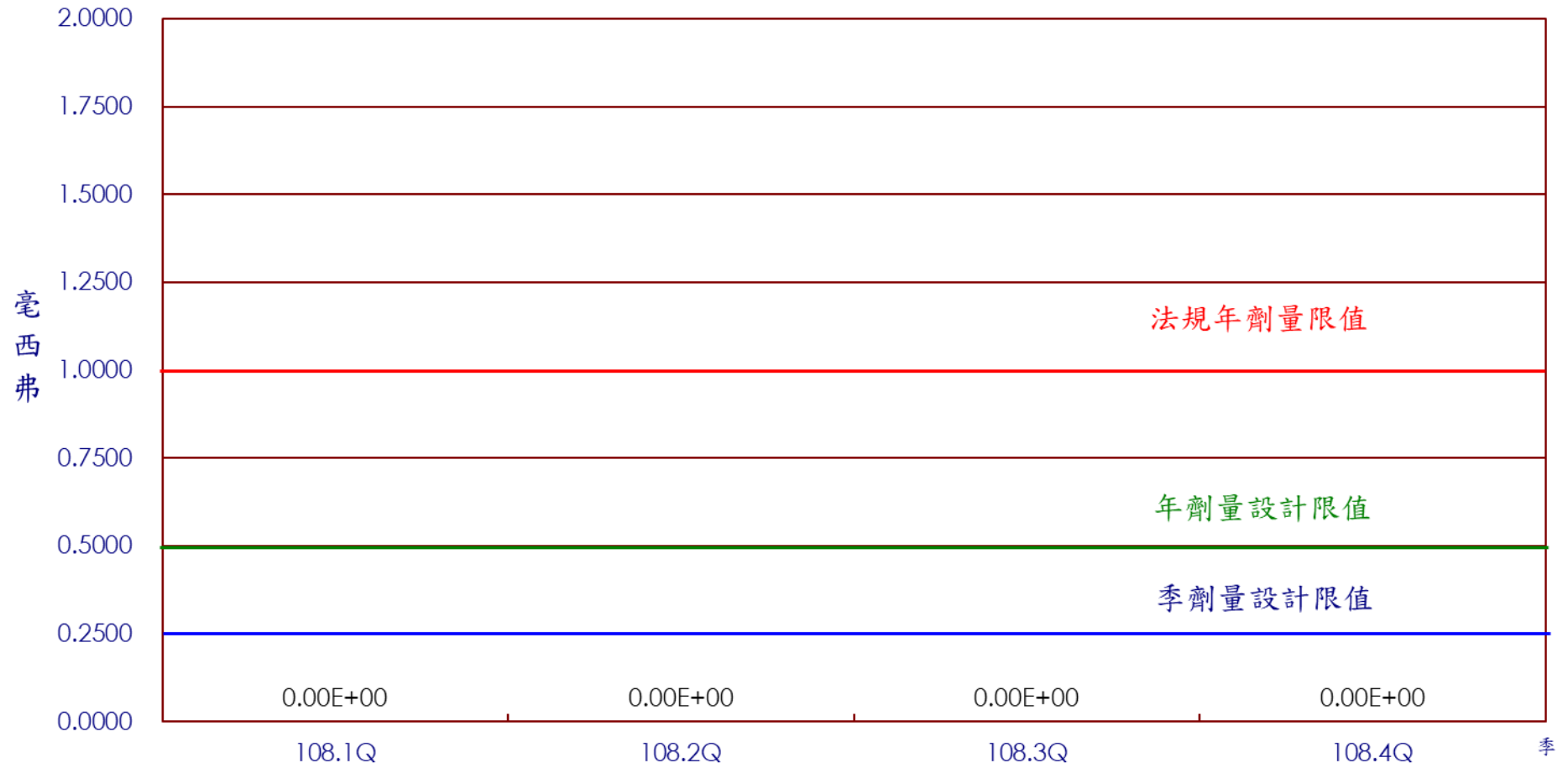
圖17 核能三廠108年第3季民眾最大個人全身劑量
