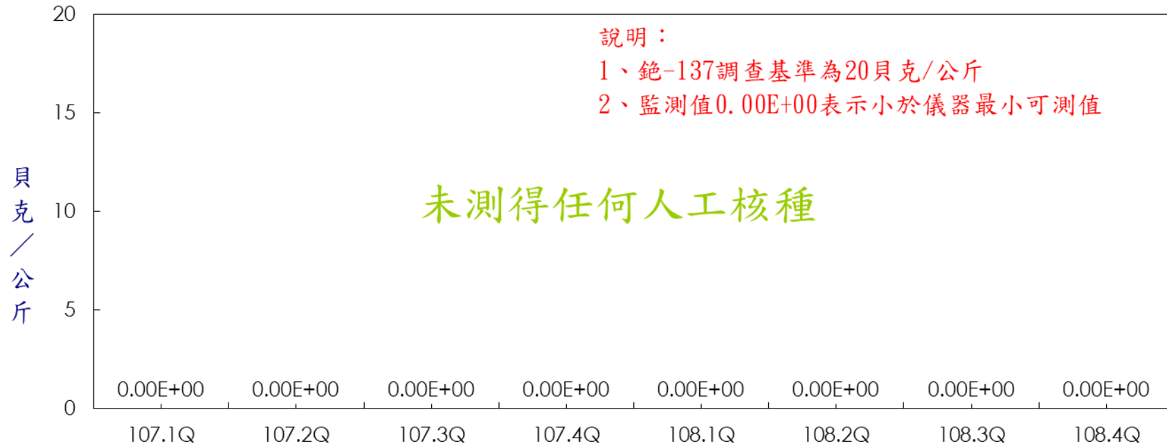
圖16 核能三廠出水口岸砂加馬能譜監測結果
