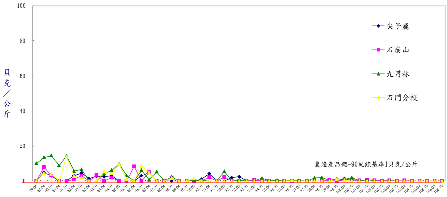
圖16 核能一廠茶葉銻-90活度歷年分析結果
