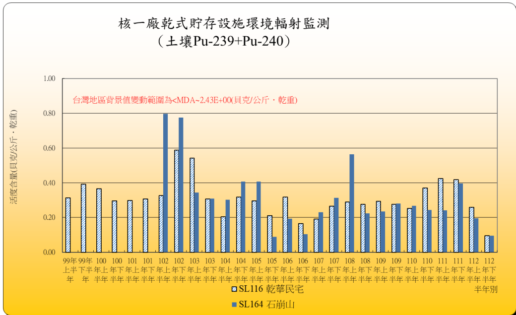
核能一廠歷年銻-238、銻-239+銻-240 監測數據趨勢如下表
