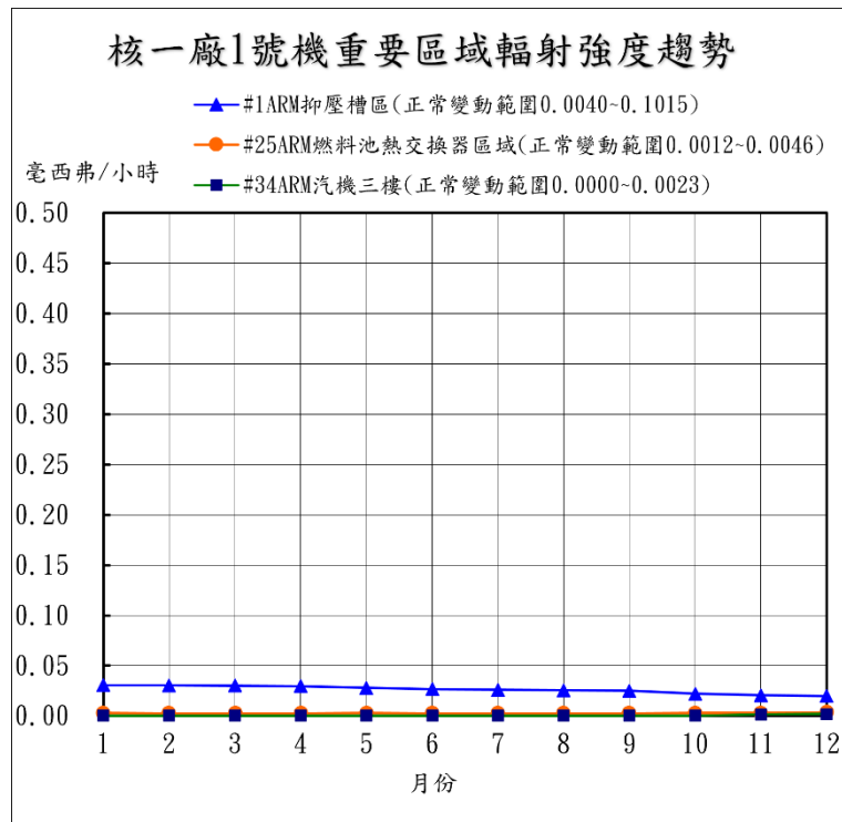
圖1 1號機重要區域輻射強度趨勢
