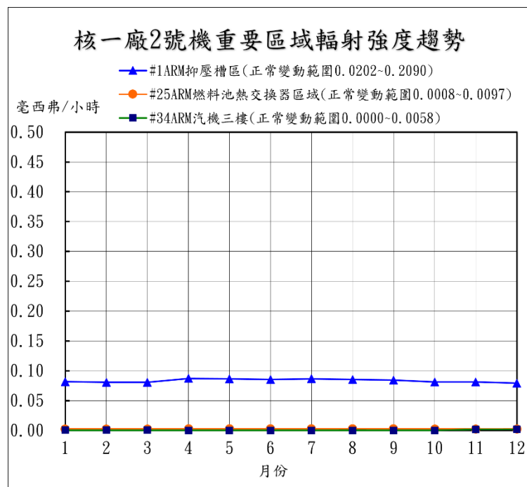
圖2 2號機重要區域輻射強度趨勢
