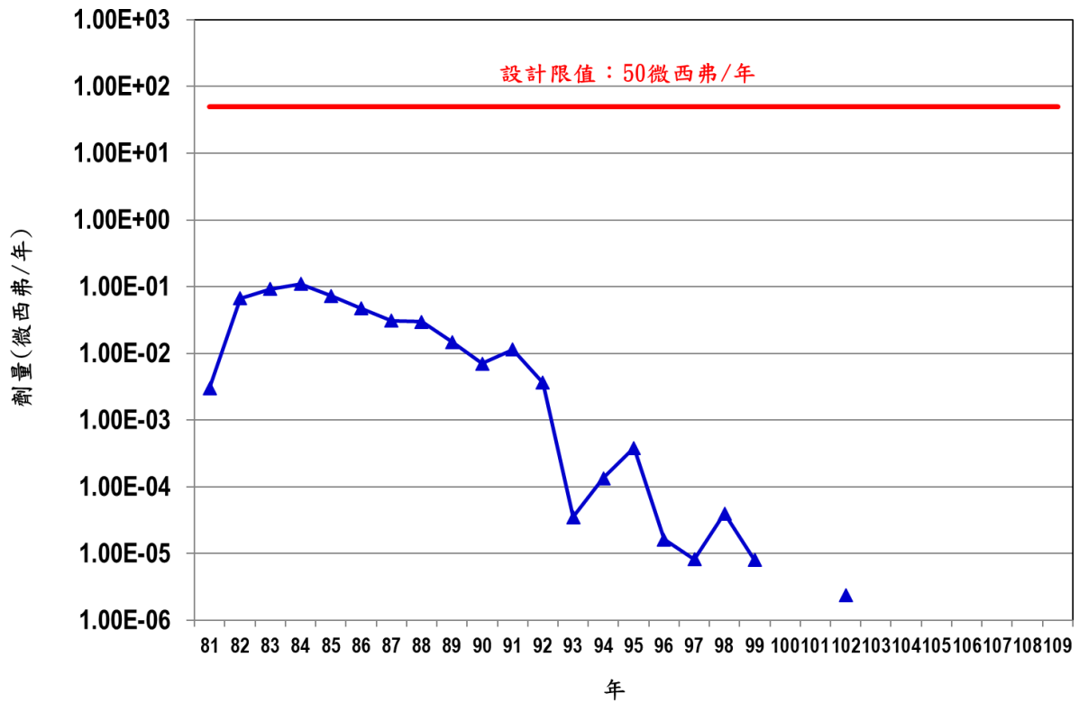
圖 5 歷年放射性廢氣排放造成關鍵群體有效劑量趨勢圖
