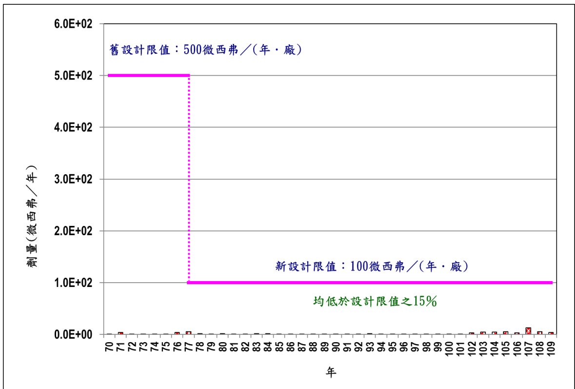
圖 11 歷年放射性廢氣排放造成關鍵群體有效劑量趨勢圖
