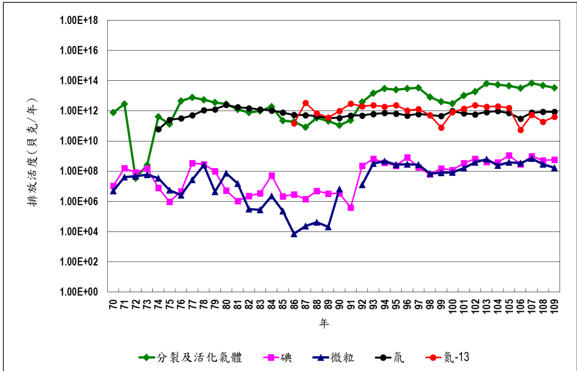
圖 6 歷年放射性廢氣排放活度趨勢圖
