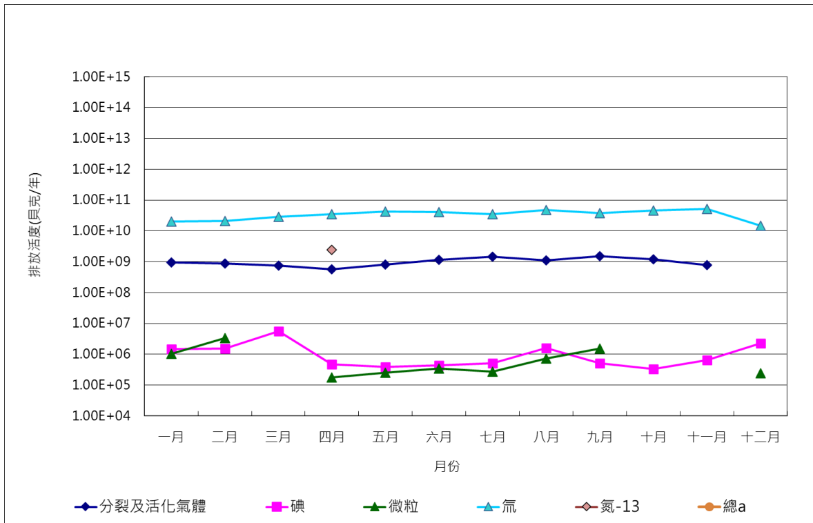
圖 9 109 年 2 號機放射性廢氣排放活度統計圖
