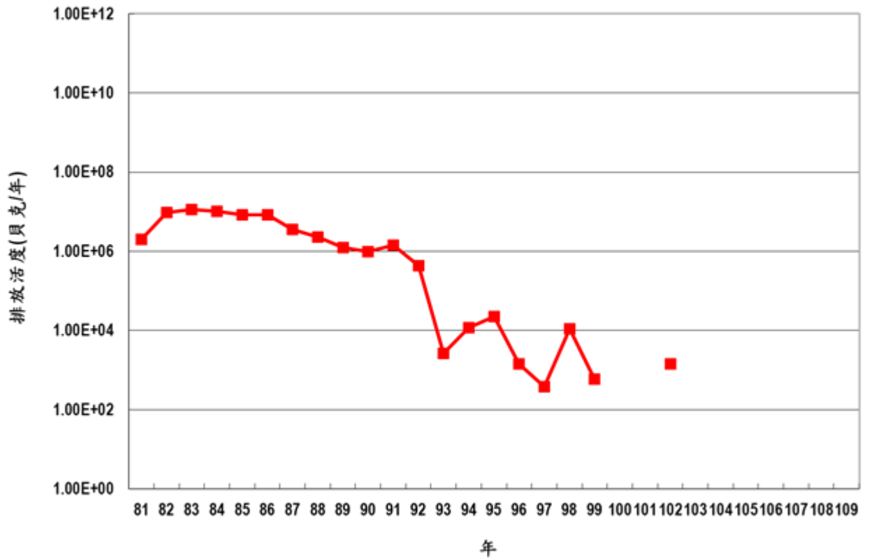
圖 3 歷年放射性廢氣排放活度統計圖
