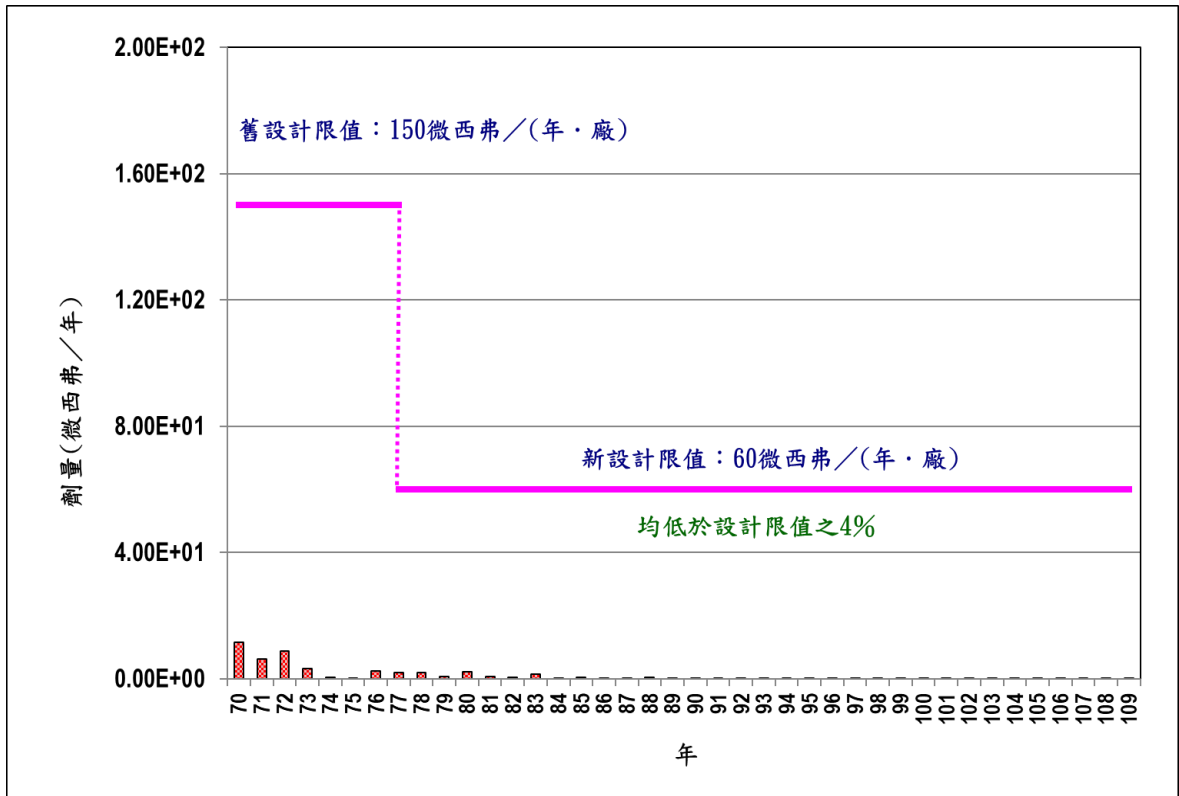
圖 12 歷年放射性廢水排放造成關鍵群體有效劑量趨勢圖
