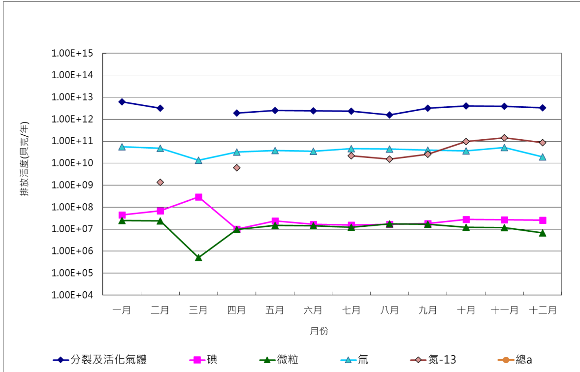
圖 8 109 年 1 號機放射性廢氣排放活度統計圖
