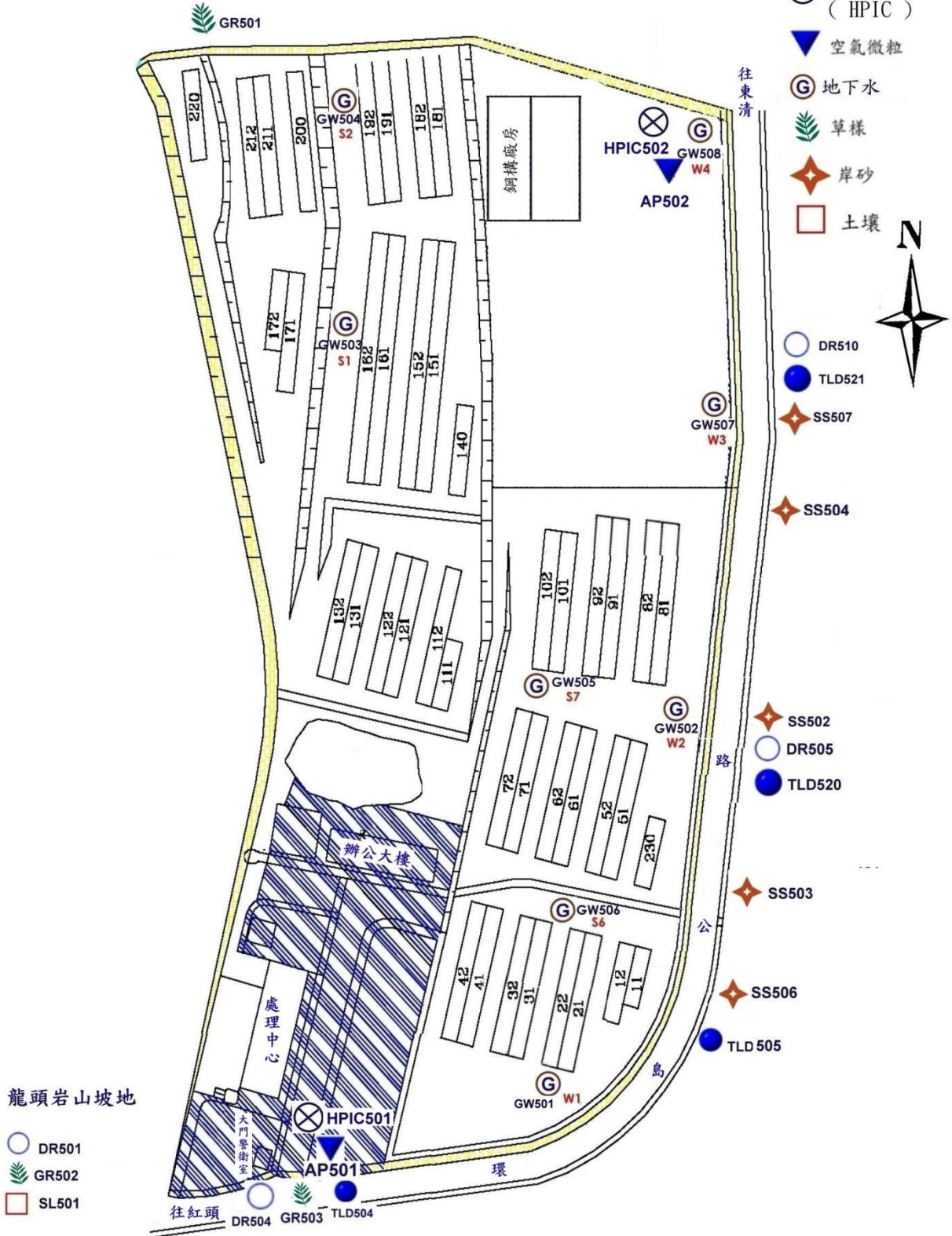
圖2 低放貯存場周邊各類試樣取樣／監測站分佈
