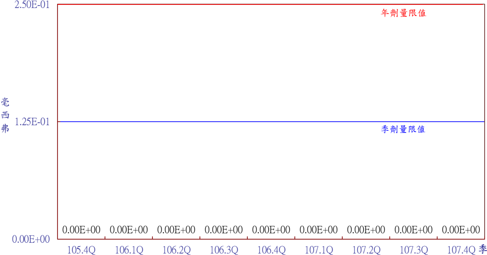
圖5 低放貯存場107年第4季民眾最大個人全身劑量
