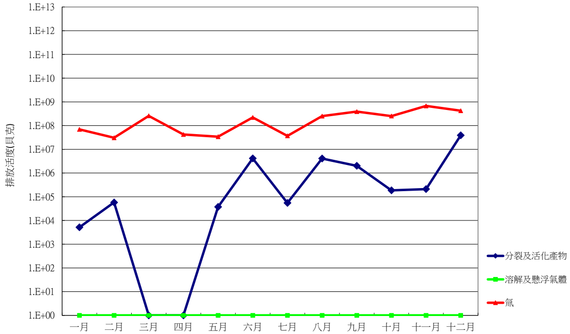
圖 8 110 年一號機放射性廢水排放活度統計圖
