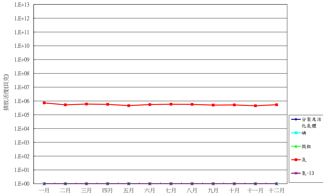
圖 7 110 年主煙囪放射性廢氣排放活度統計圖
