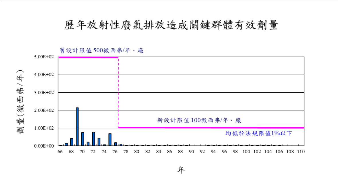
圖 10 歷年放射性廢氣排放造成關鍵群體有效劑量趨勢
