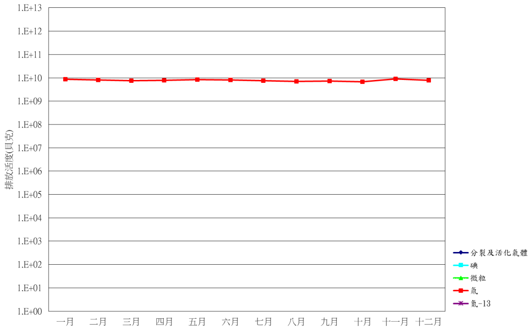
圖 6 109 年二號機放射性廢氣排放活度統計圖
