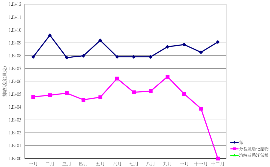
圖 8 109 年一號機放射性廢水排放活度統計圖
