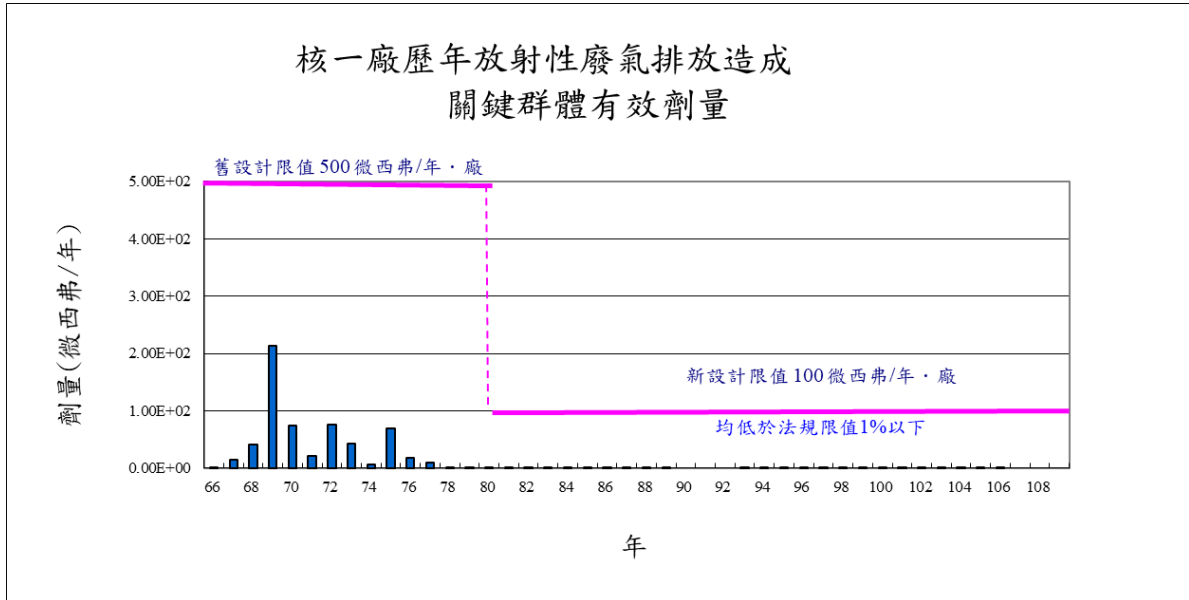
圖 10 歷年放射性廢氣排放造成關鍵群體有效劑量趨勢
