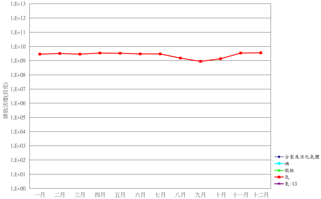
圖 5 109 年一號機放射性廢氣排放活度統計圖
